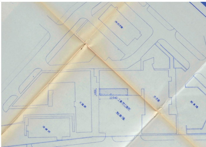
配置図
