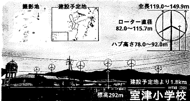
※地平線と山の標高より風力発電 149.9mを想定。イメージです。 ※建設予定地、機体トレース…2020年7月 日立サステナブル エナジー株式会社配布資料より引用
