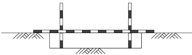
路面復旧工
