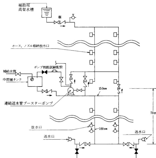
図19-1 加圧送水装置の設置例
