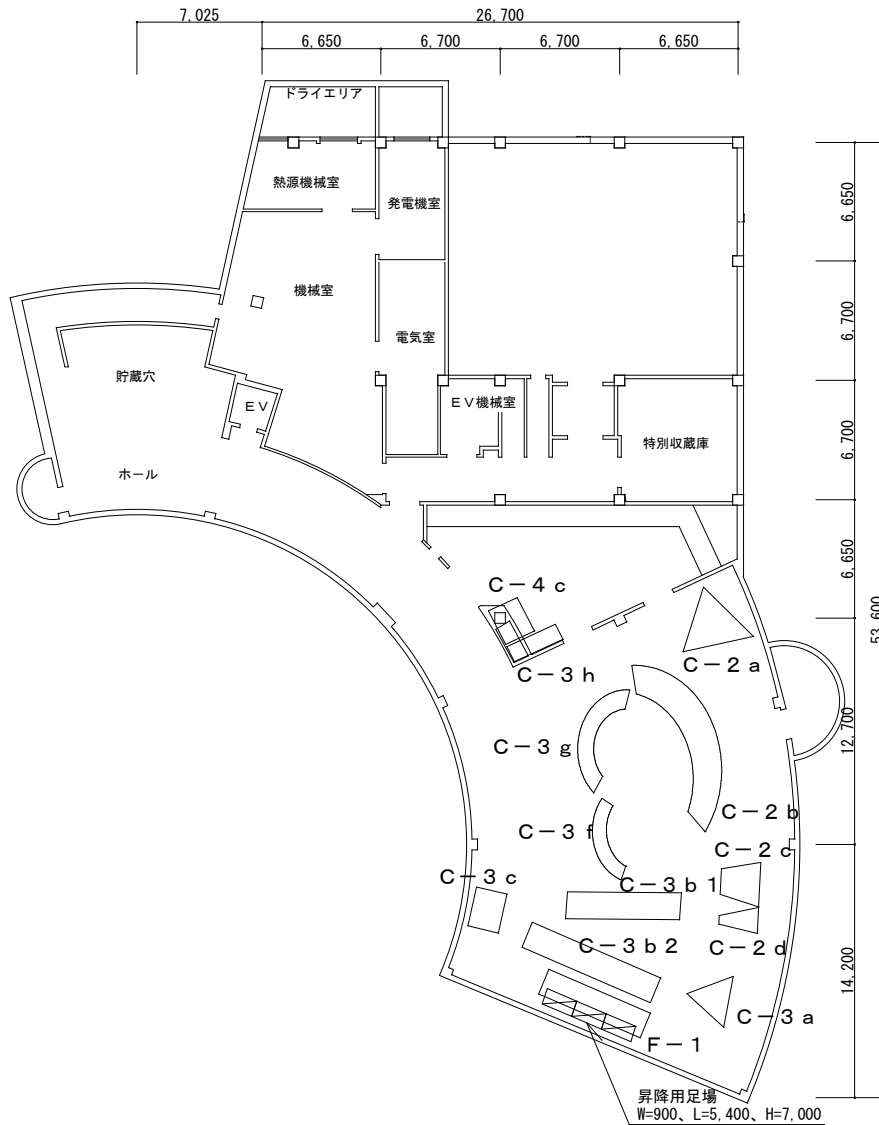
地下1階平面図 S=1/300
