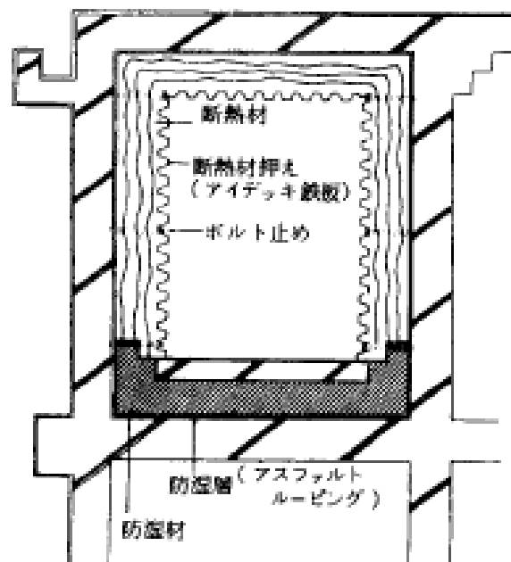
図6—2 冷凍室等断熱処理施工例
