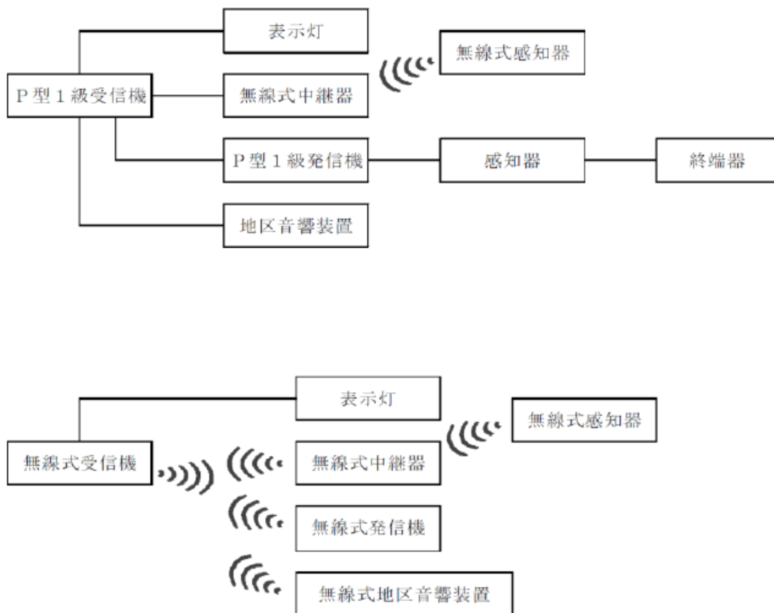
図10の 2 - 1 無線式自動火災報知設備の構成図例
