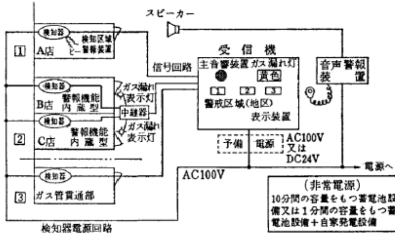
図11-10 ガス漏れ火災警報設備のシステム構成図
