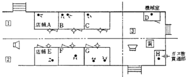
図11-11 警報装置の設置例
