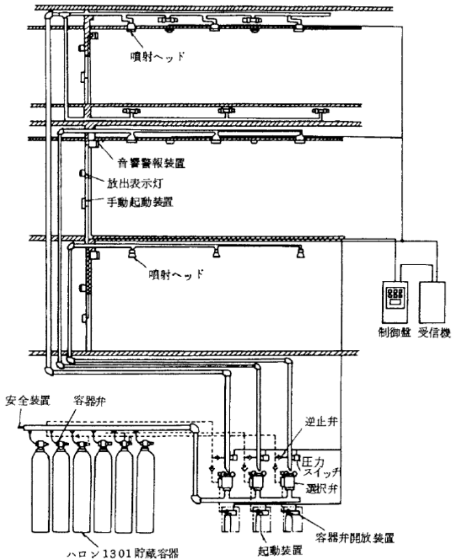
図7-1 ハロゲン化物消火設備の構造図例
