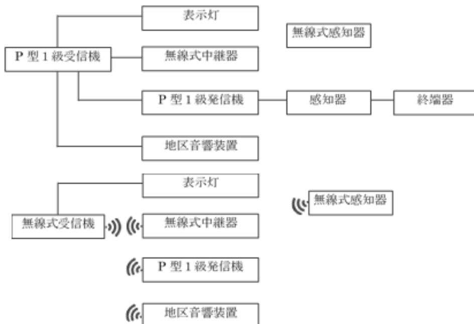
図10-2 無線式自動火災報知設備の構成図例
