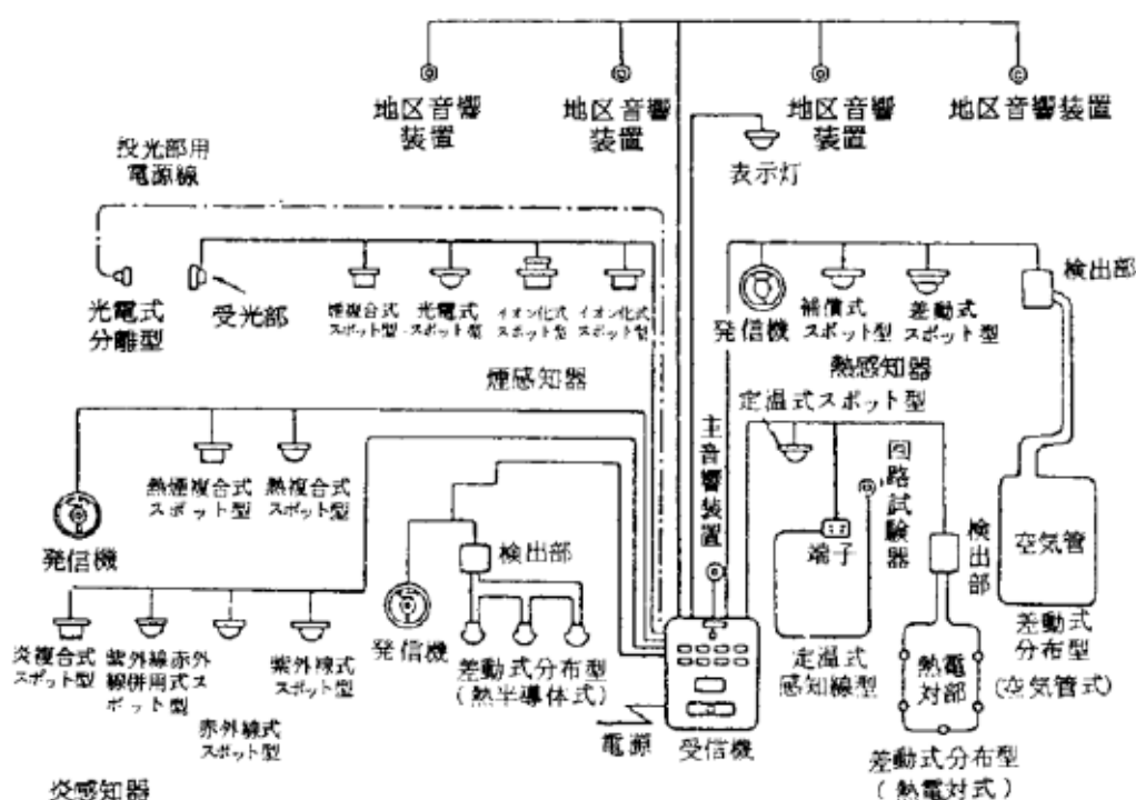
図10—1 自動火災報知設備の構成図例
