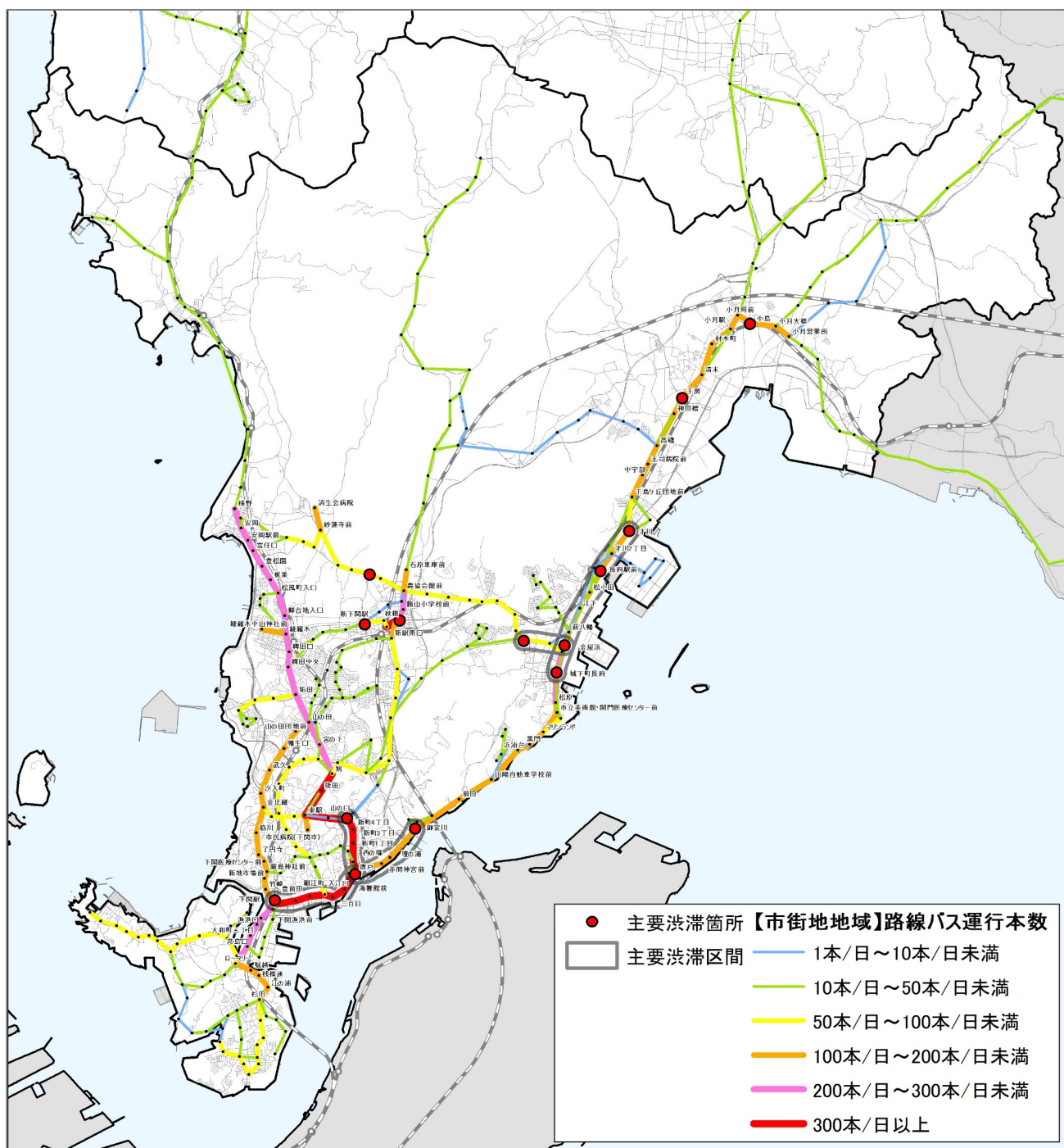
図 2.3 路線バス運行本数及び主要渋滞箇所
