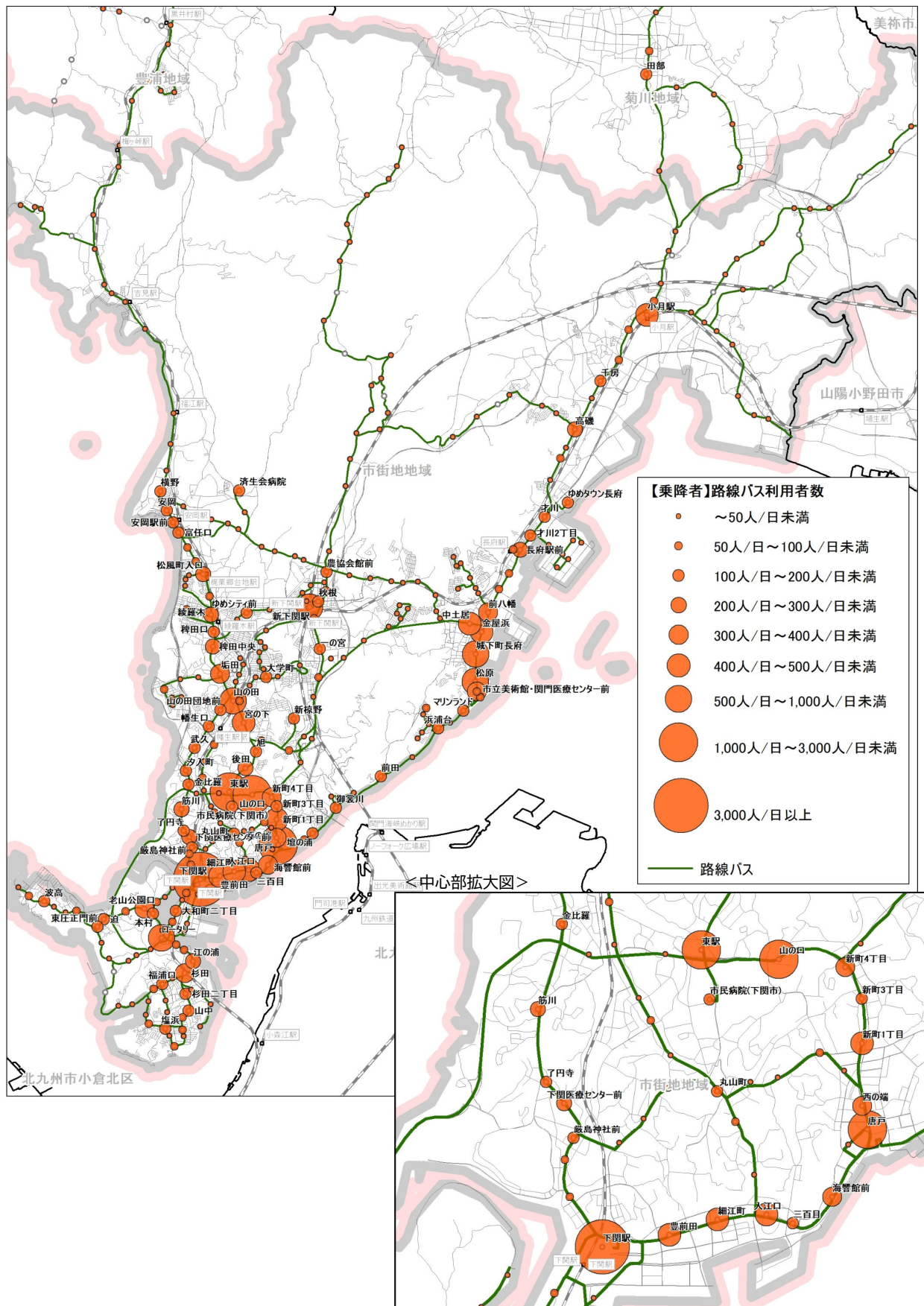
図 2.21 バス停別利用者数(平日) (市街地拡大)
