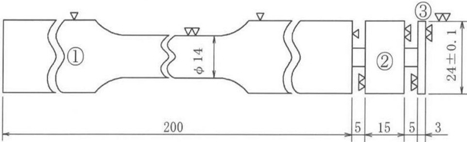
① 引張試験片 ② 硬さ試験片・黒鉛球状化率判定試験片 ③ 腐食試験片
