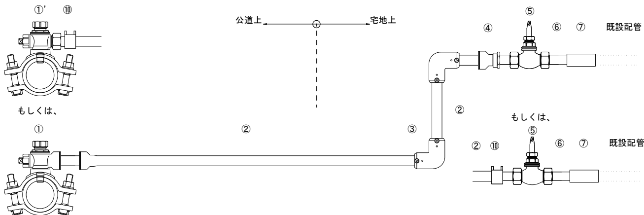
本管分岐 ~ 宅内止水栓 配管図
