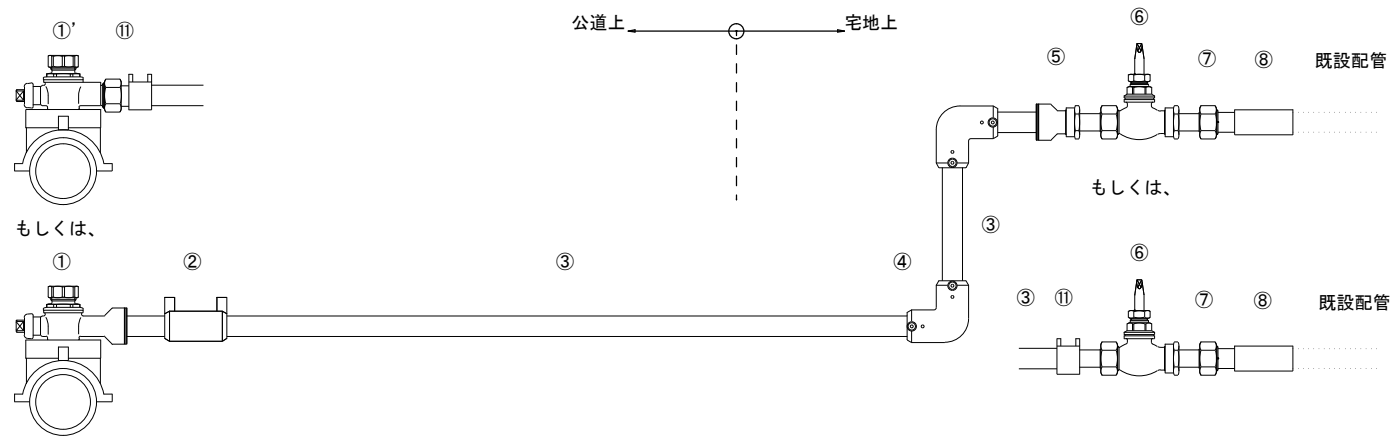
本管分岐 ~ 公道ボール止水栓 配管図
