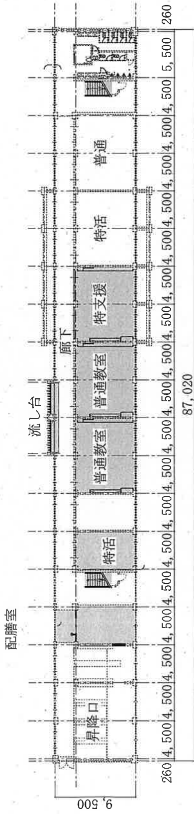
普通教室棟 1階平面図
