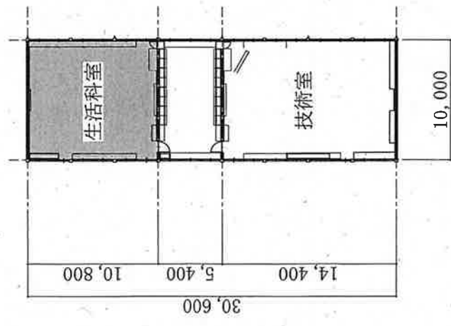
特别教室棟 平面图
