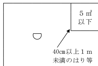
差動式、補償式、定温式 各スポット型の場合
