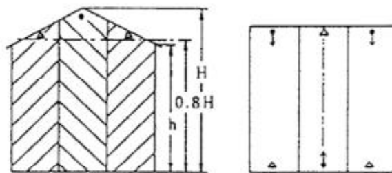
●→ は送光部、△は受光部 斜線は監視区域を表す。 (以下の図において同じ。)
