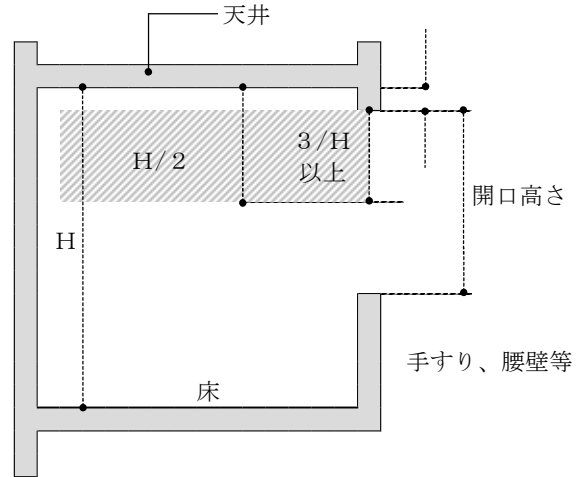
【外気流通場所が1/3以上の高さ（例）】
