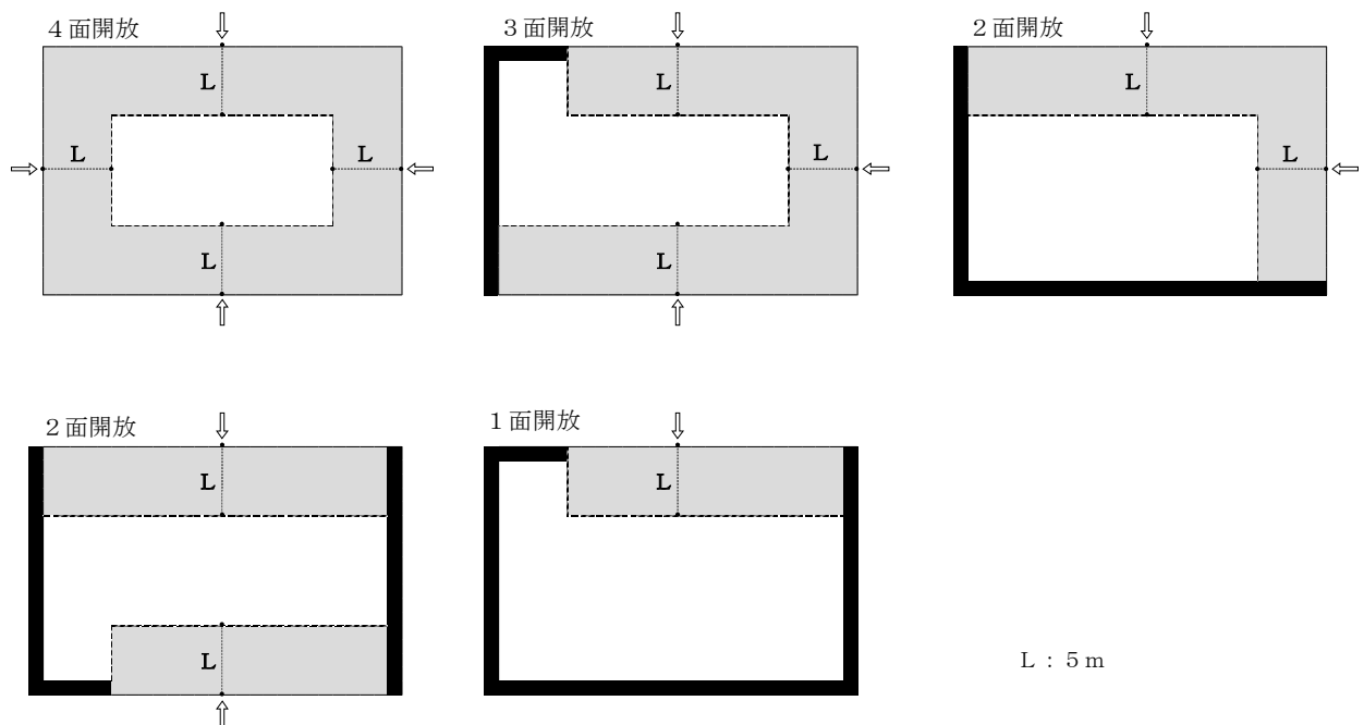
【直接外気に面するそれぞれの部分から5m未満の場所（例）】
