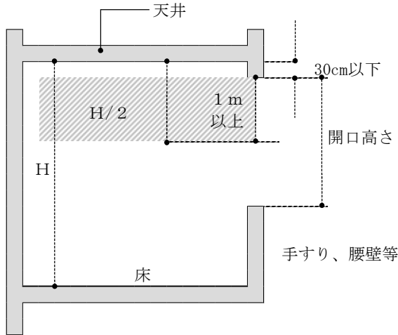
【外気流通場所が1 m以上の高さ（例）】
