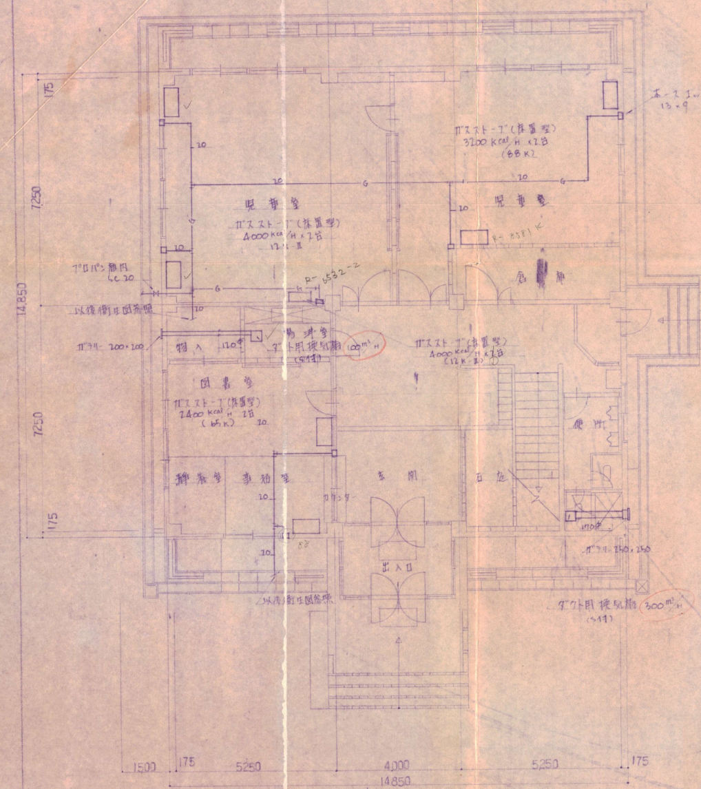
1階平面図 1:100
