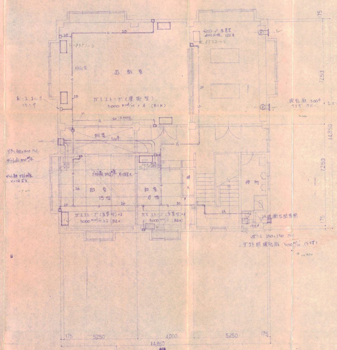
2階平面図 1:100
