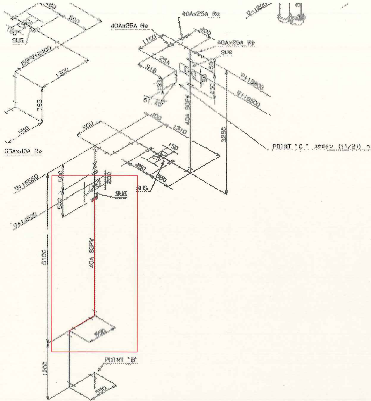
消化棟 配管図
