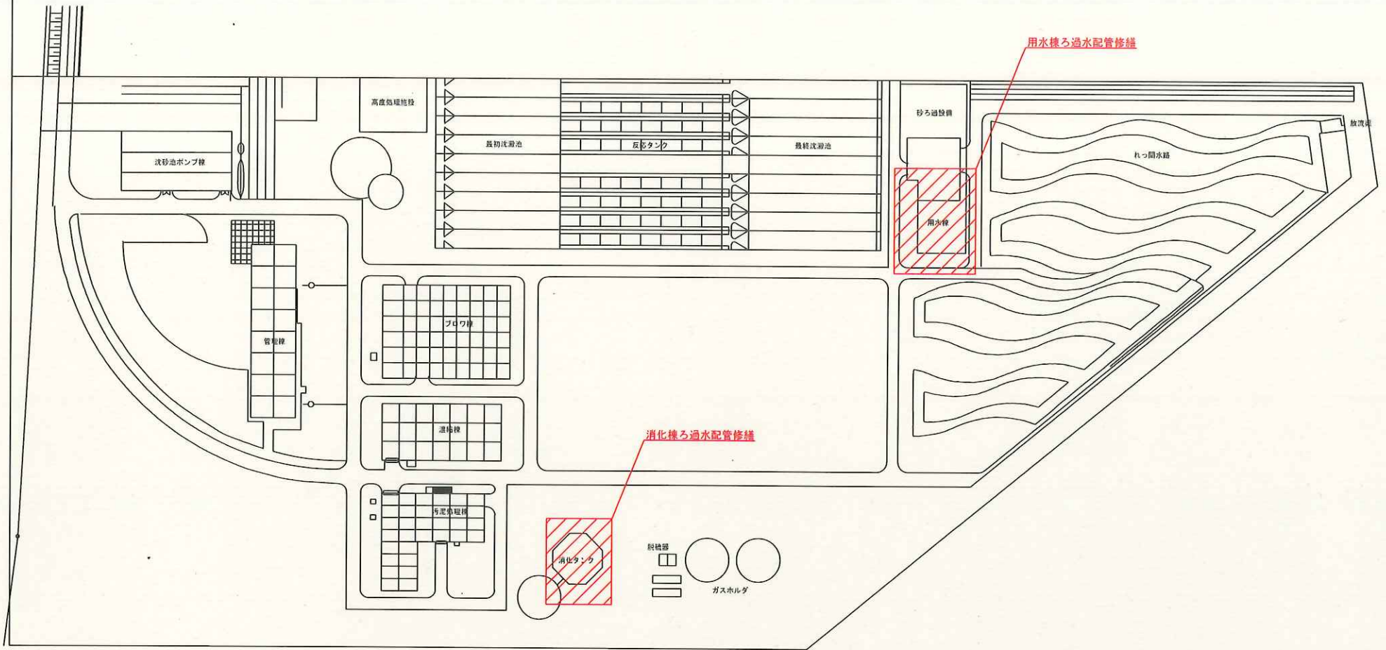
山陽終末処理場 平面図
