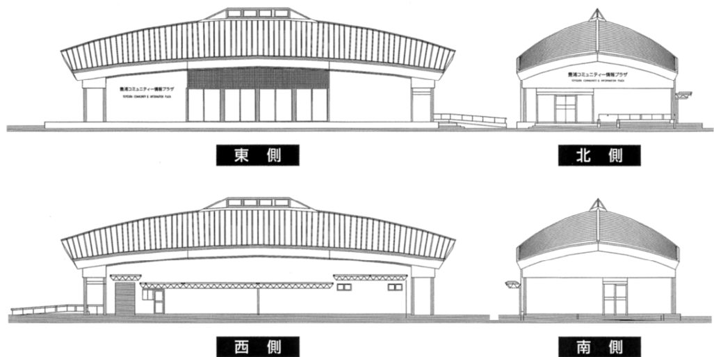
情報プラザ本体立面図
