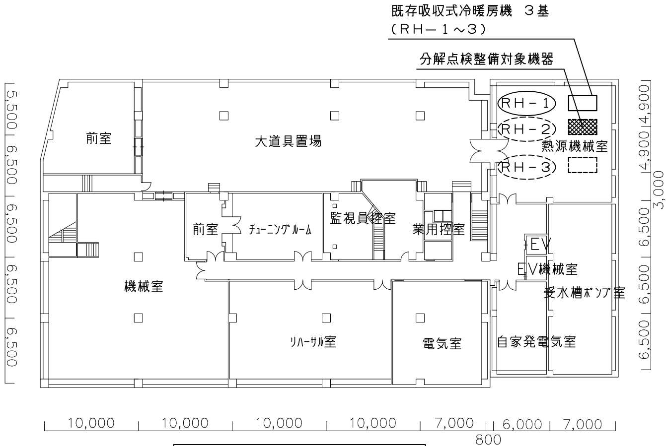
地階平面図 S：1／400
