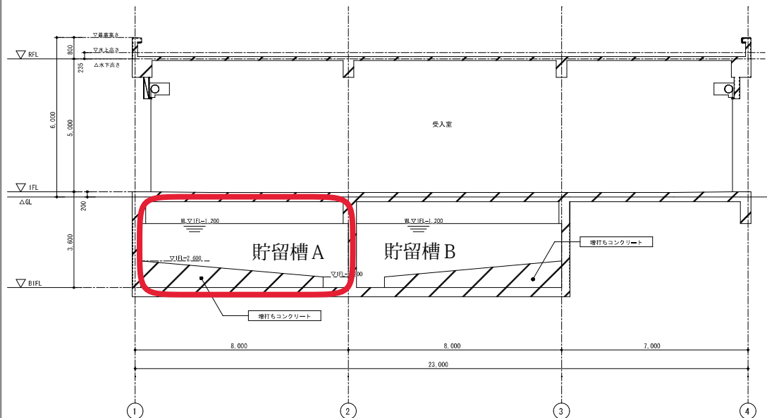
断面図C 1:100
