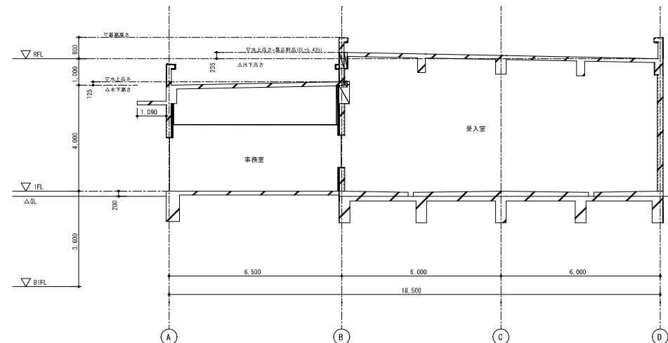
断面図B 1:100
