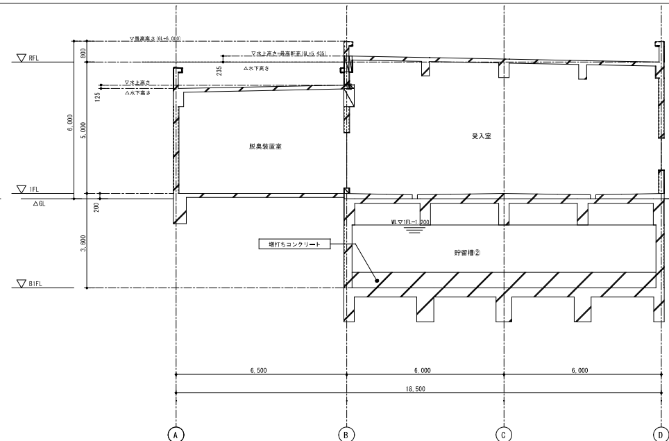
断面図B 1:100
