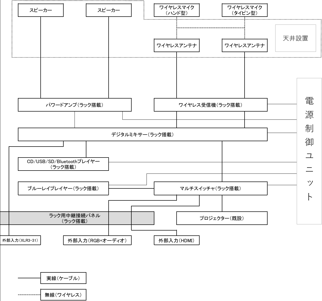
機器接続図
