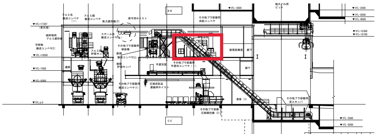
処理棟 断面図
