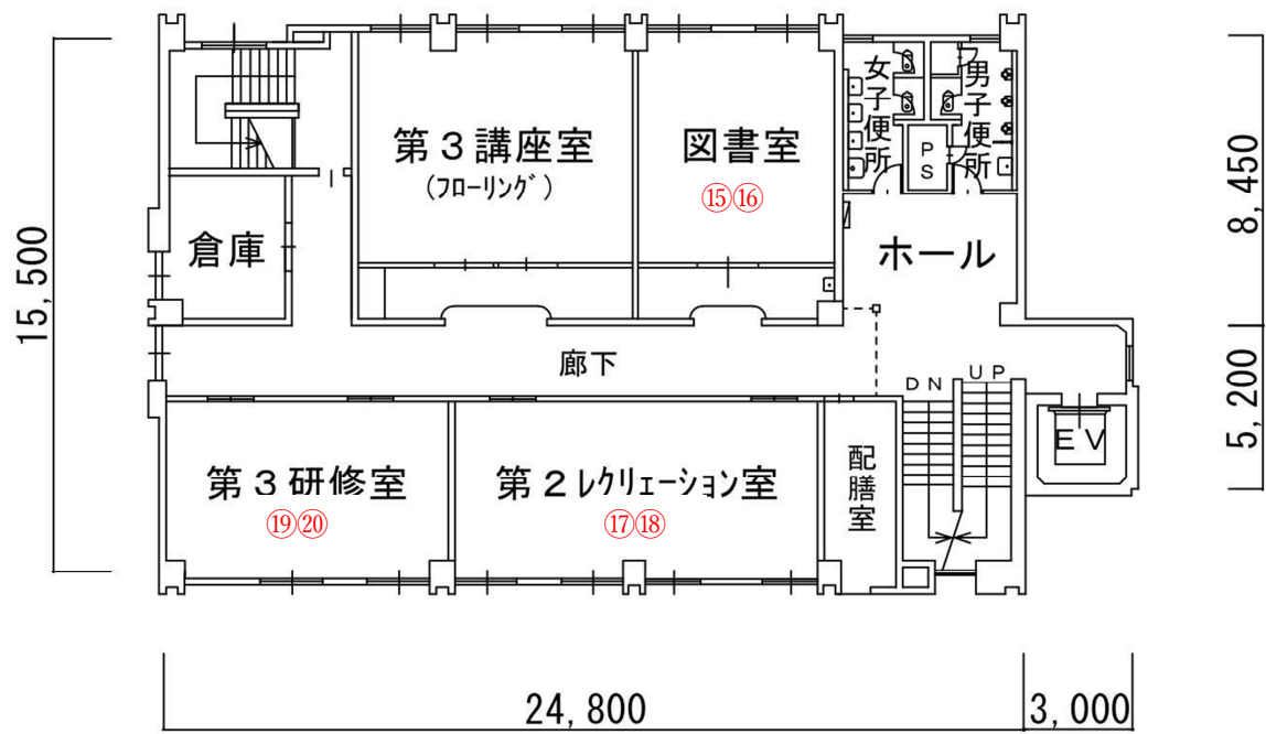
4階平面図
