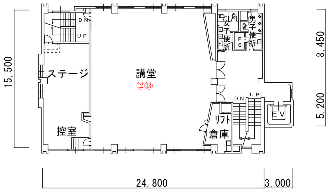
3階平面図
