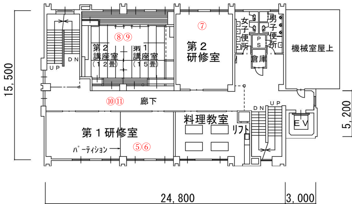
2階平面図
