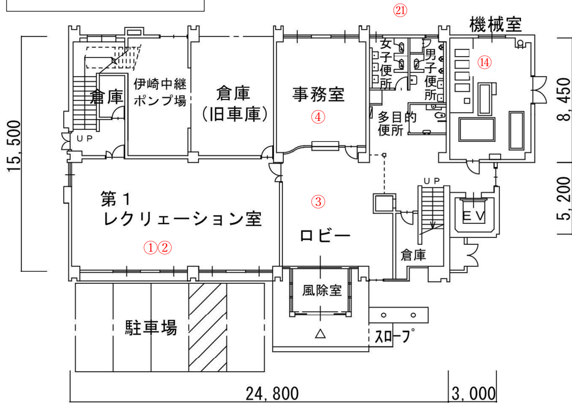
1階平面図
