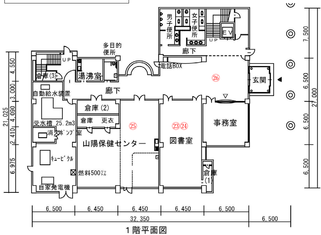
下関市立長府東公民館平面図
