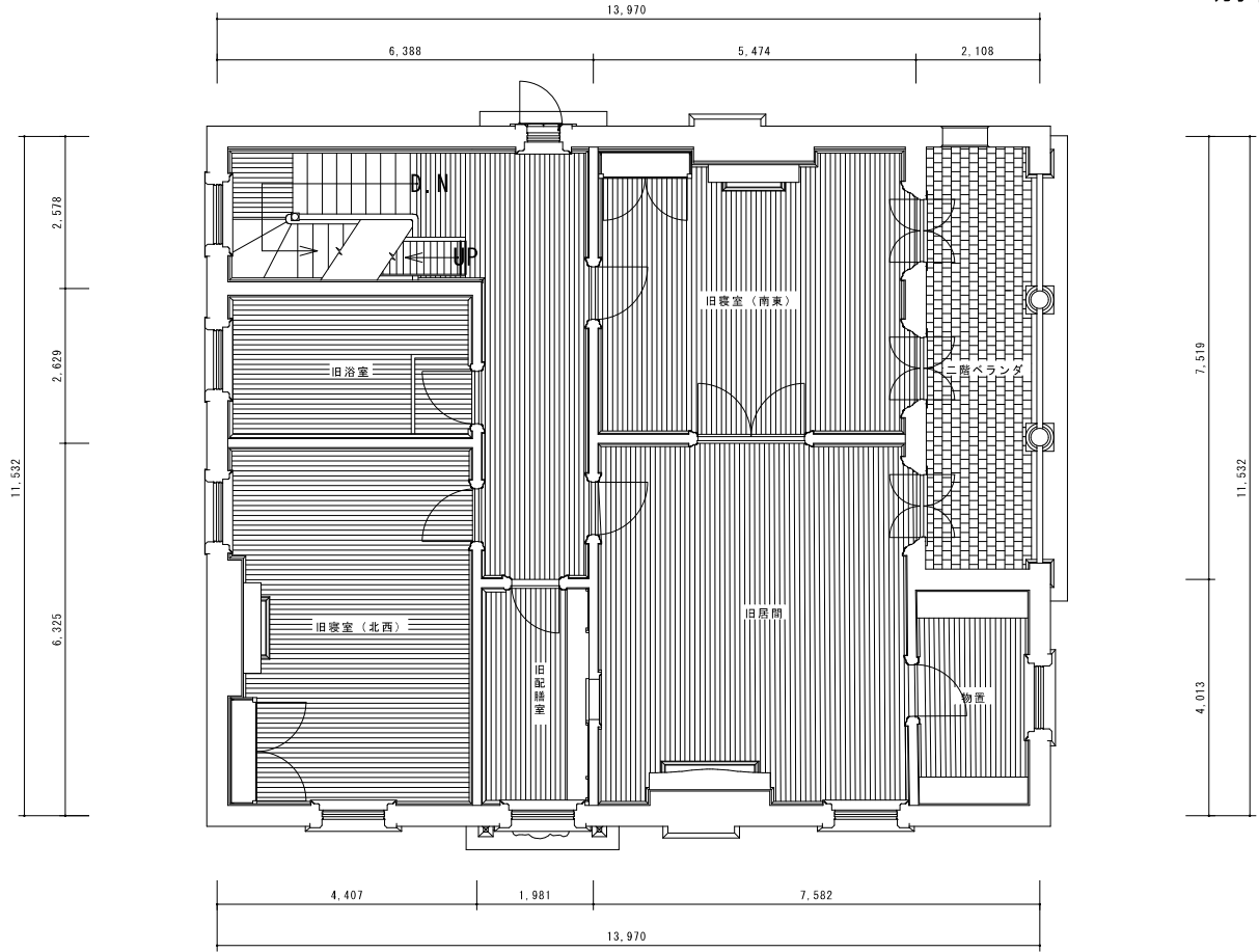
本館 2 階平面図
