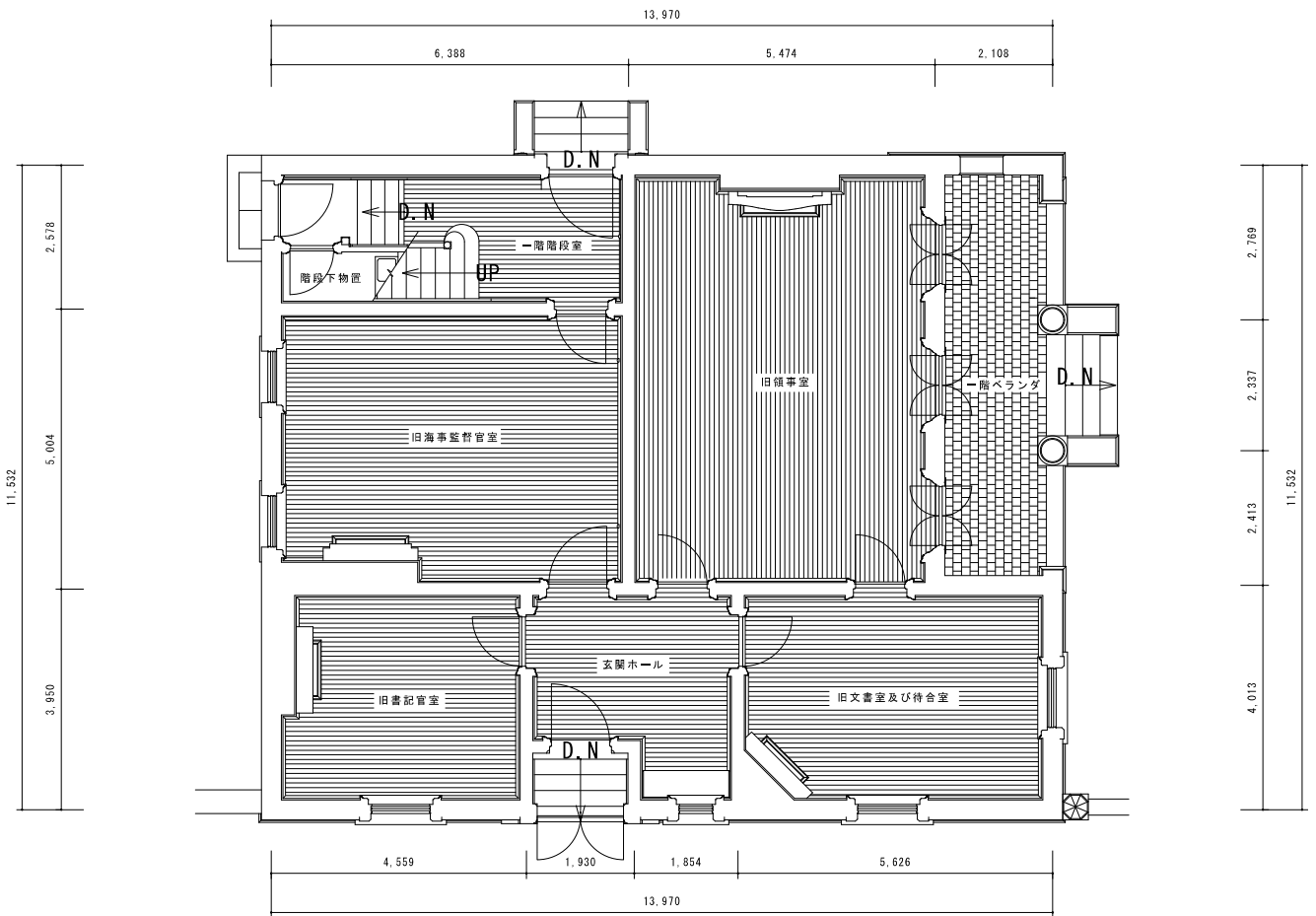
本館 1 階平面図
