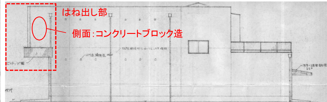
図2 立面図(側面)
