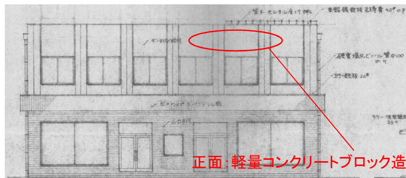
図1 立面図(正面)
