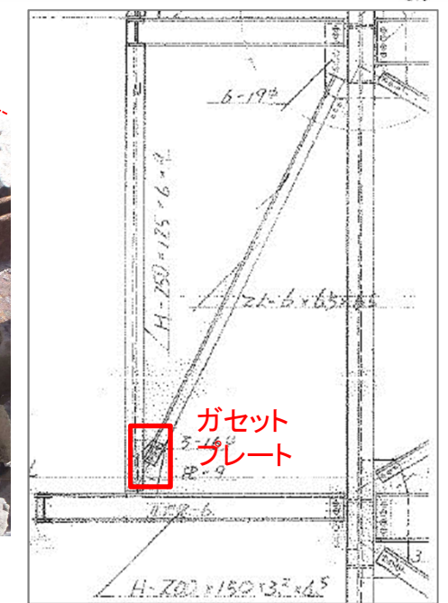
図4 2階はね出し部断面図
